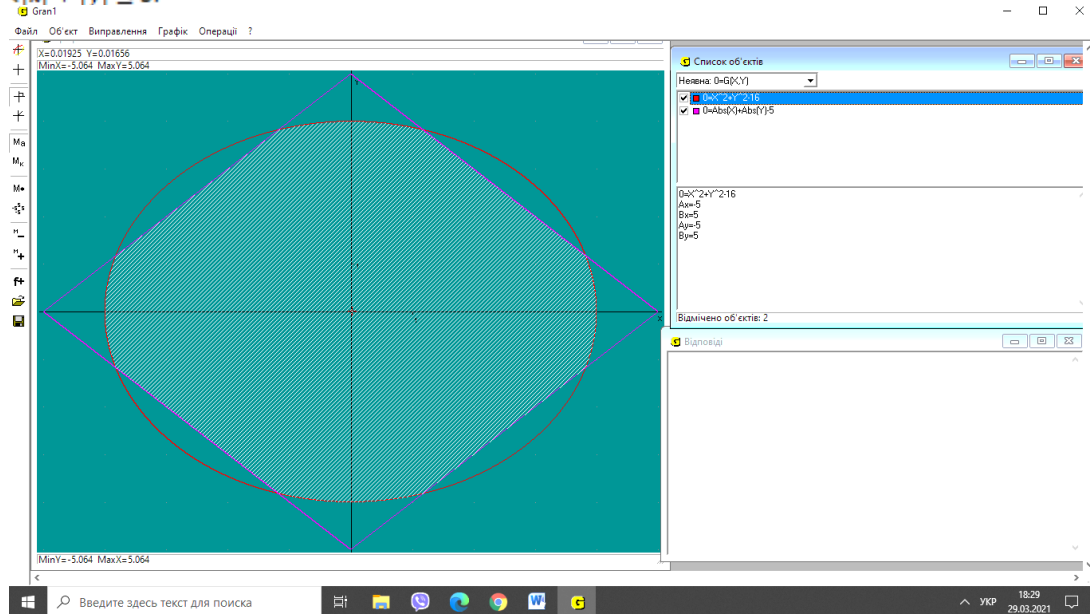
Рис. 2 Графіки функцій x^2 + y^2 \leq 16 та |x| + |y| \leq 5 та у GRAN-1
