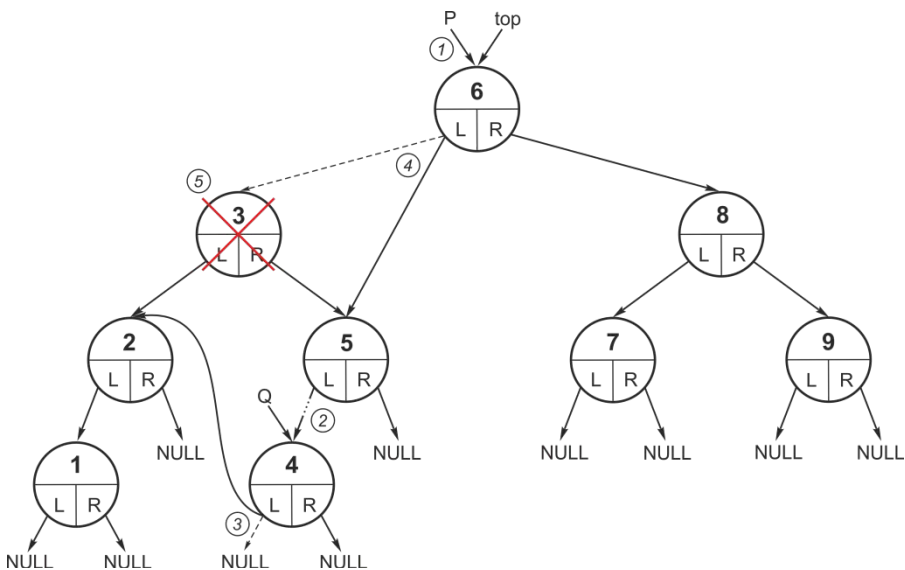
Рис. 35. Видалення вузла із заміною на праве піддериво
