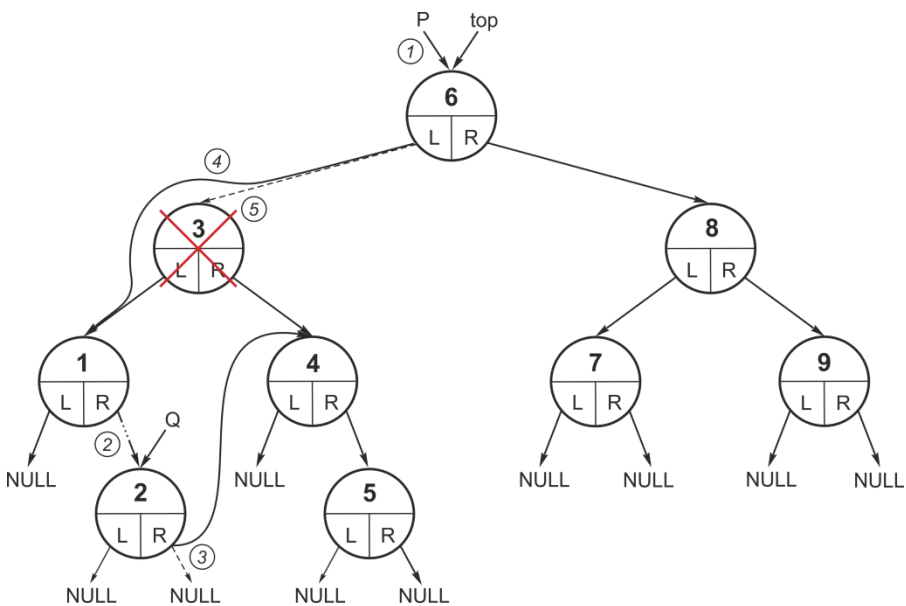
Рис. 34. Видалення вузла із заміною на ліве піддереву
