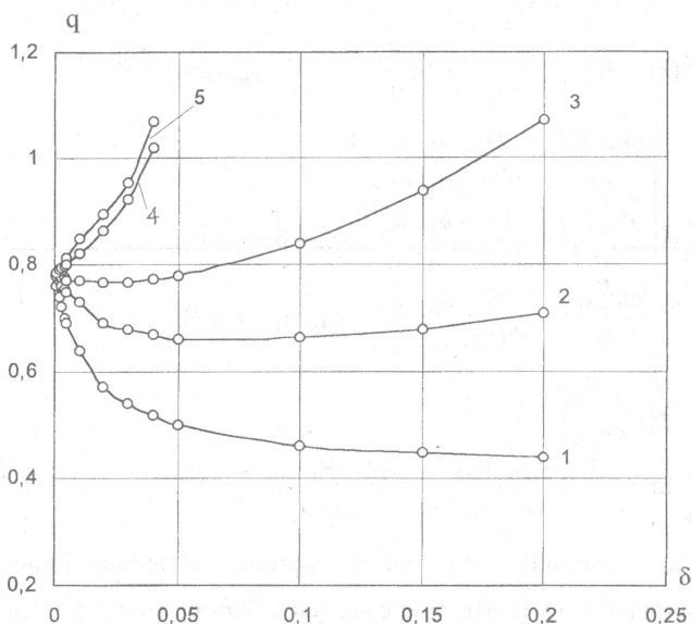
Рис.1. Графік залежності q = q(\delta) при k_\phi = 2; 5; 10; 50; 100 (відповідно криві 1-5).
