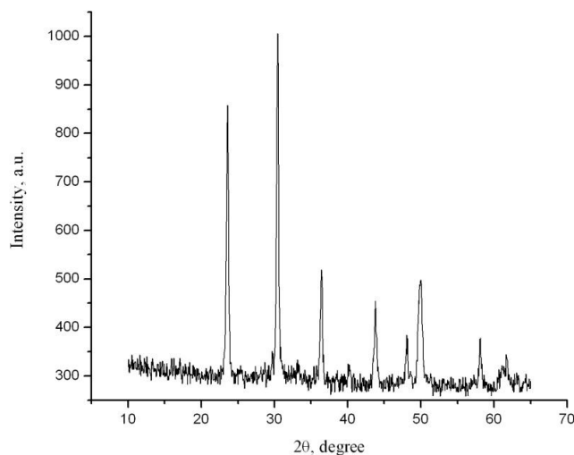
Рис. 2. Дифрактограма дрібнодисперсного порошку, отриманого на протягом 4 год за температури електроліту 25 °С
