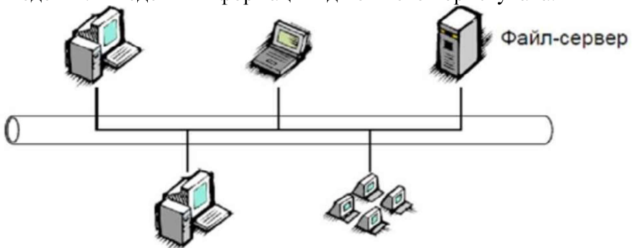
Рисунок 2.2 Файл-серверна архітектура
