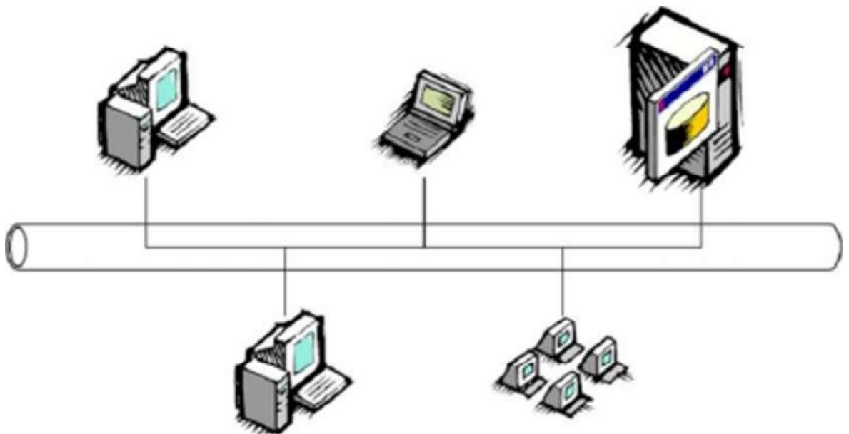
Рисунок 2.4 Архітектура клієнт-сервер
