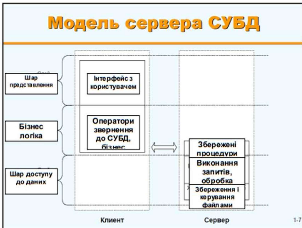
Рисунок 2.5 Архітектура клієнт-сервер
