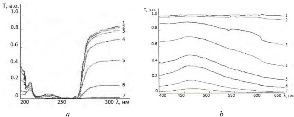
Рис. 2. (а) Спектри пропускання в ближній УФ області в процесі полімеризації 0,01М розчину аніліну під дією ПДСА в 0,5 М сульфатній кислоті.
