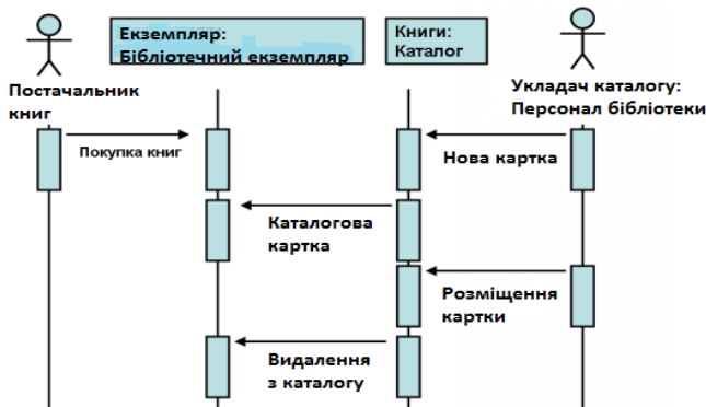
Рис.2.17. Діаграма послідовності
