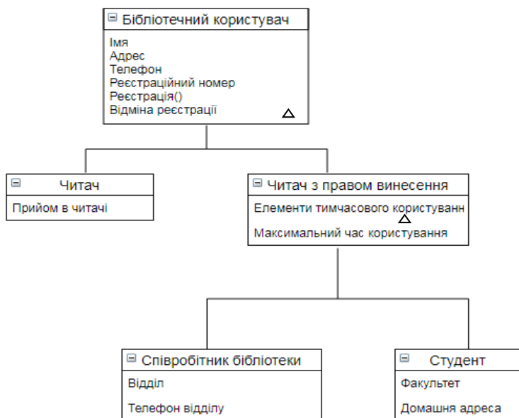
Рисунок 30 – Моделі наслідування
