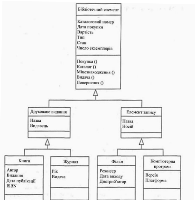
Рисунок 29 – Модель класів
