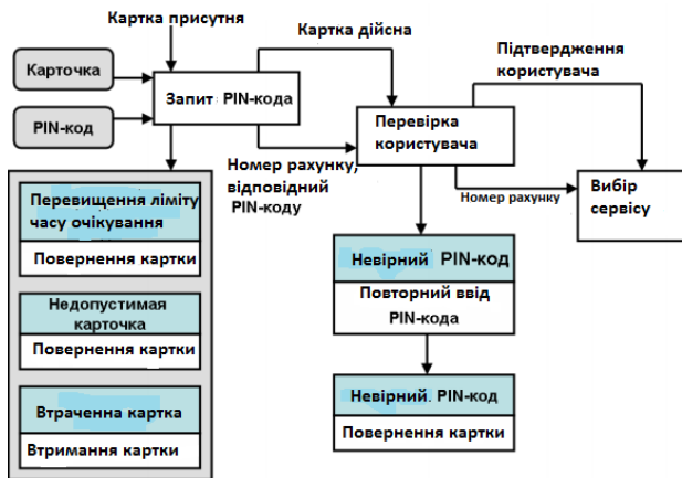
Рис.2.15. Діаграма сценаріїв
