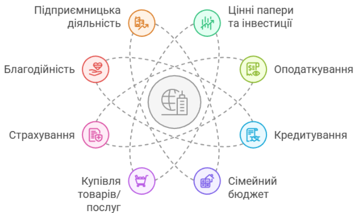
Рис. 1. Комплекс сфер і процесів застосування математичних знань
