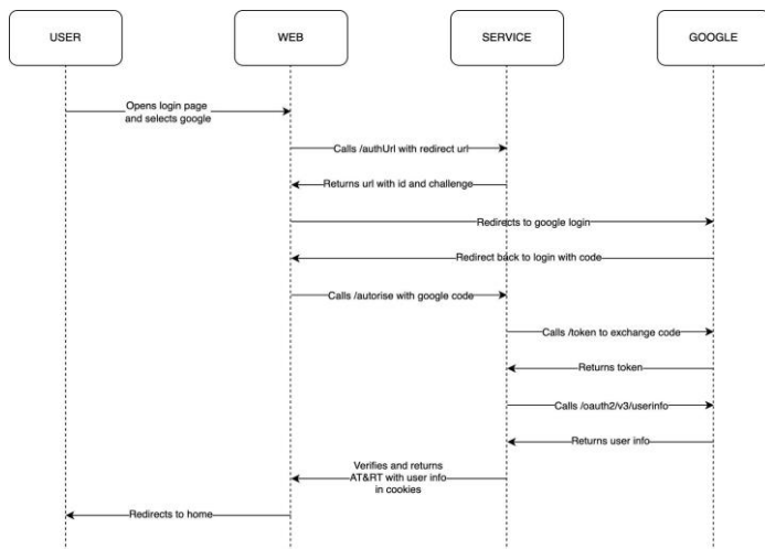
Рис. 1 Діаграма взаємодії з Google OAuth 2.0
