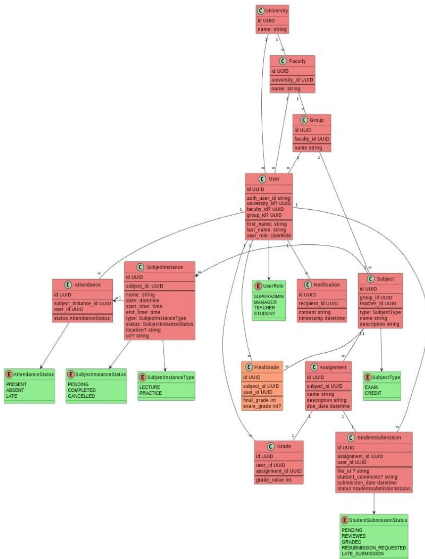
Рис. 1. Модель бази даних
