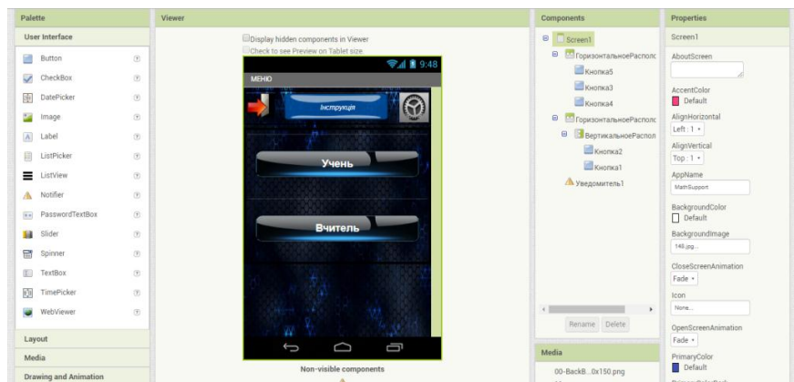
Рис. 2. Конструктор компонентів в App Inventor [2]
