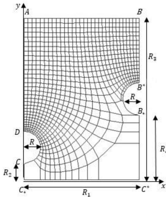
Рис.1. Область фільтрації G_z
