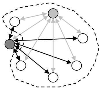
Рис.1. Структурний граф
