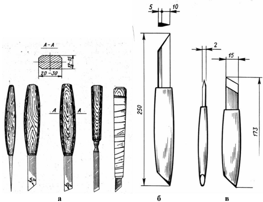
а – стамески й ножі, б – богородський ніж, в – ніж косяк
