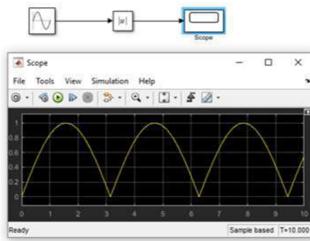
Рис. 2 Використання блоку Abs
