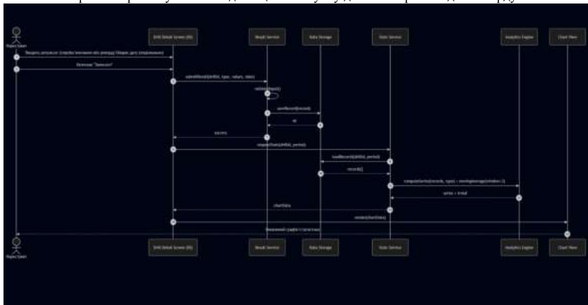
Рис. 1. Діаграма послідовностей застосунку
