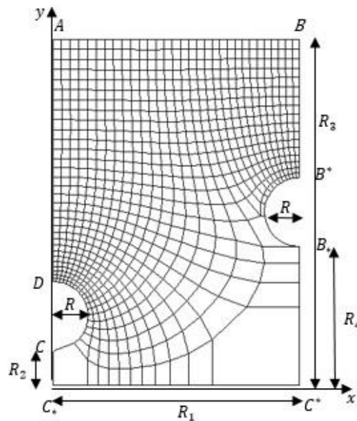
Рис.1 – Схематичне зображення фільтраційного процесу в горизонтальному дренажі
