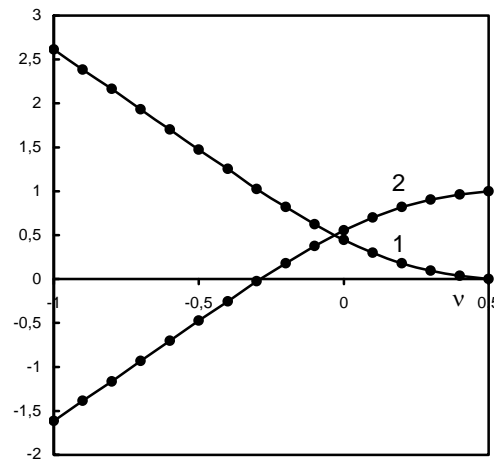
Рис. 1. Залежність коефіцієнта C (1) і 1 - C (2) від величини \nu .
