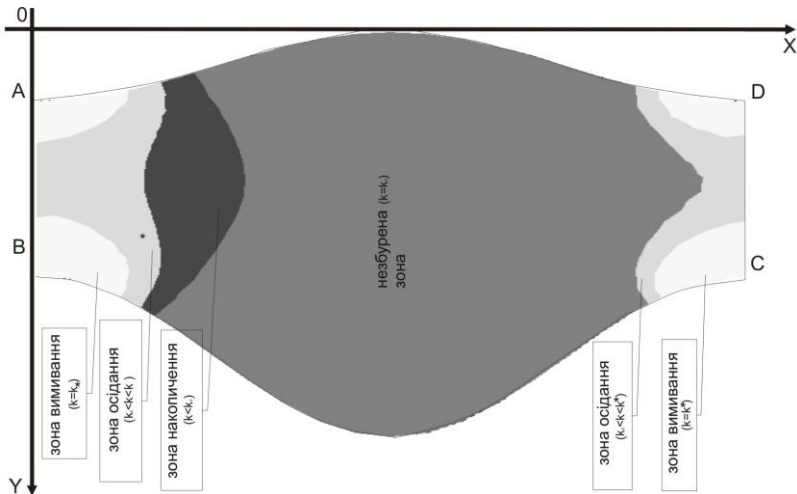
Рис. 3. Зони збурення згідно (11)
