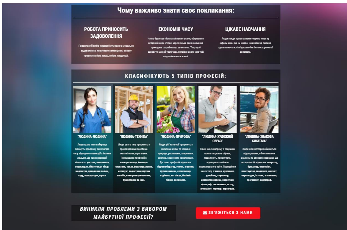
Рис.1. Головна сторінка
