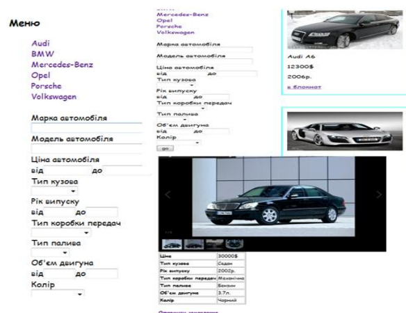
Рис. 1. Користувацька частина
