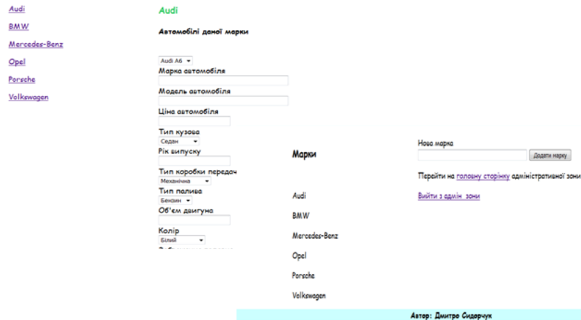
Рис. 2. Адміністративна частина
