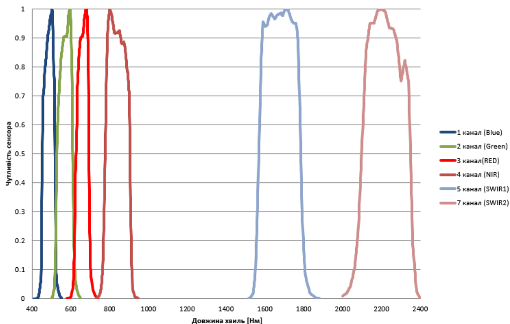
Рис. 2.2. Спектральне охоплення сенсора TM супутників Landsat-4,5
