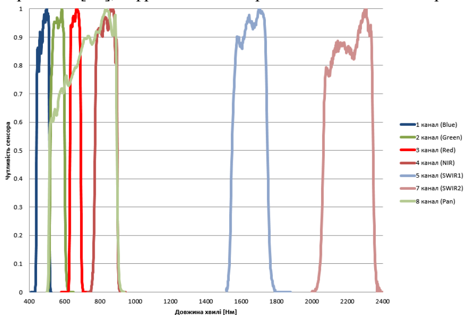
Рис. 2.3. Спектральне охоплення сенсора ETM+ супутника Landsat-7
