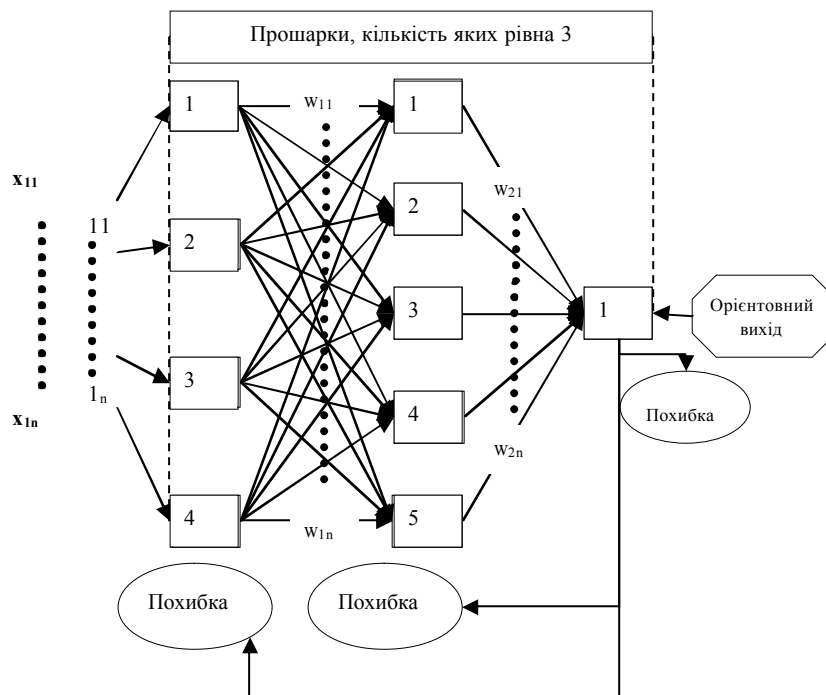
Рис.1 Вигляд нейронної мережі зворотнього поширення
